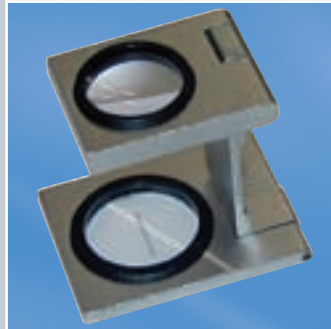
Präzisions-Fadenzähler aus Stahl, mit Strichplatte (Teilung 1/10 mm), 8-fache Vergrößerung, aplanatisch
