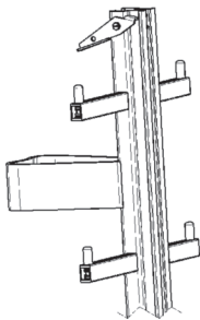
Abb.7 Bsp. Al- Einholmleiter mit beweglichem Endanschlag
